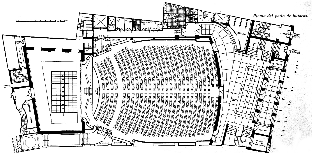
Plantas del teatro Albéniz. R.N.A., Año X, nºs 104-105, agosto-septiembre 1950.
