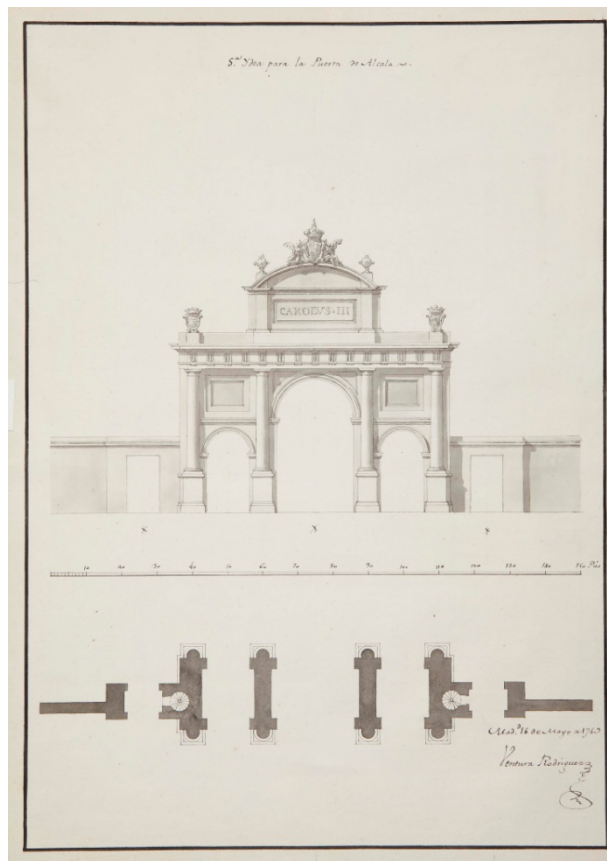
Fig. 109- Ventura Rodríguez: 5. a Ydea para la Puerta de Alcalá, 1769. Museo de Historia de Madrid.
