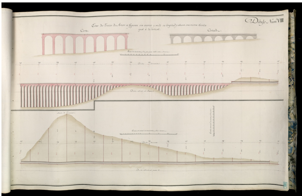
Fig. 117- Ventura Rodríguez: Delineación del acueducto de la ciudad de Pamplona, Dibujo Numº VIII, 1782 . Archivo Municipal de Pamplona / Colección de Mapas, Planos y Dibujos.
