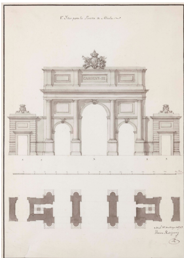
Fig. 106- Ventura Rodríguez: 1. a Ydea para la Puerta de Alcalá, 1769. Museo de Historia de Madrid.
