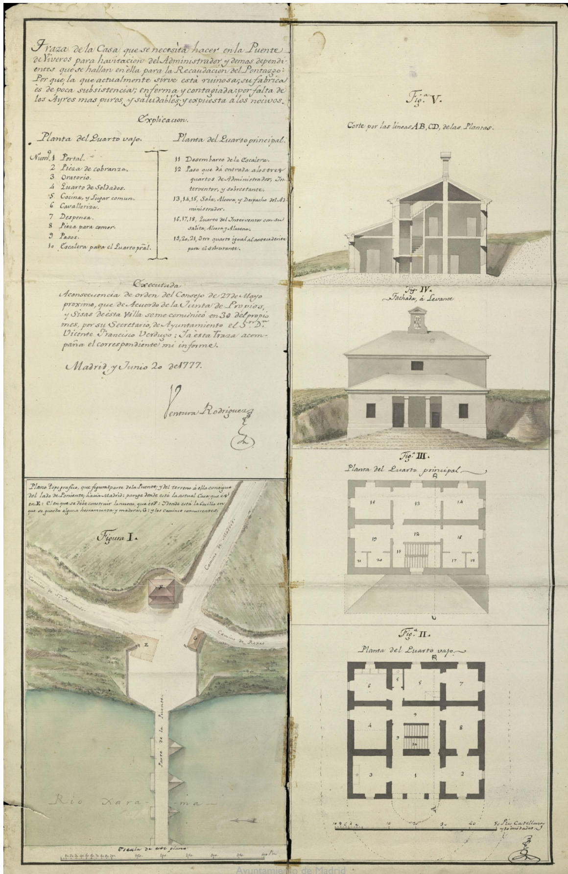
Fig. 101- Ventura Rodríguez: Traza de la Casa que se necesita hacer en la Puente de Viveros para habitación del administrador y demás dependientes que se hallan en ella para la Recaudación del Pontazgo, 1777.
