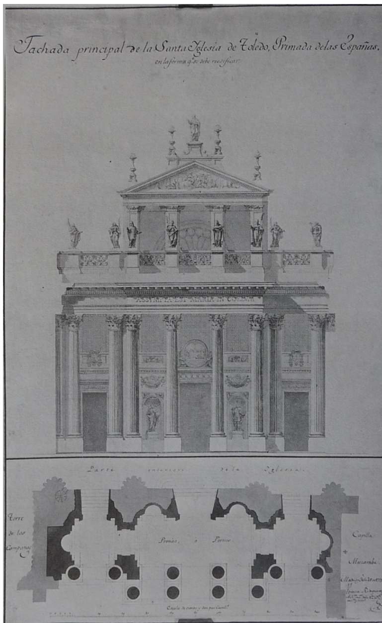
Fig. 71- Ventura Rodríguez: “ Fachada principal de la Santa Iglesia de Toledo, Primada de las Españas, en la forma q.ª se debe reedificar ”, 1773. Excmo. Cabildo de la Catedral Primada de Toledo (publicada en El arquitecto D. Ventura Rodríguez, 1717-1785 ).
