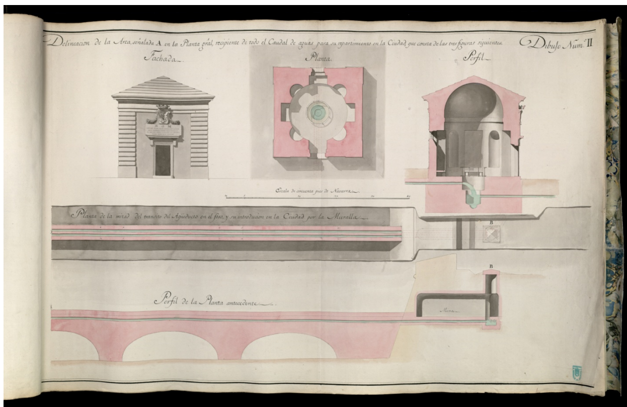
Fig. 116- Ventura Rodríguez: Delineación del acueducto de la ciudad de Pamplona, Dibujo Num o II , 1782. Archivo Municipal de Pamplona / Colección de Mapas, Planos y Dibujos.
