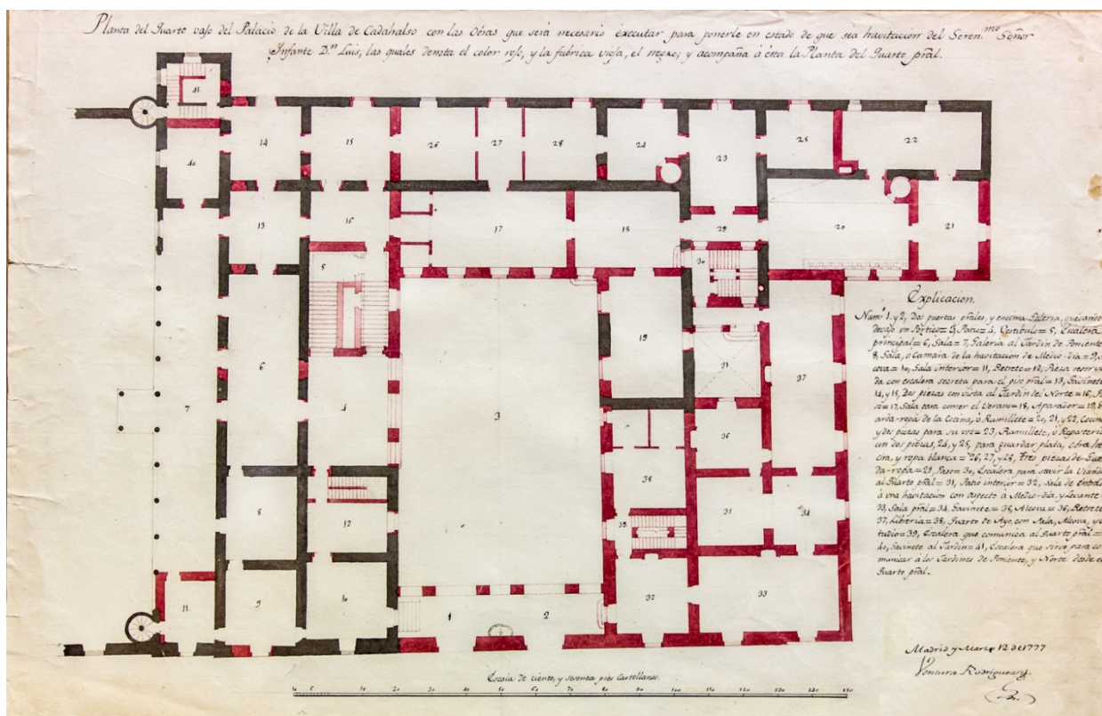
Fig. 23- Ventura Rodríguez: “Planta del Quarto bajo del Palacio de la Villa de Cadahalso con las obras que será necesario executar para ponerle en estado de que sea havitación del Seren.º Señor Ynfante D.º Luis”, 1777. Colección particular.
