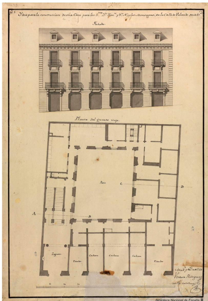
Fig. 5- Ventura Rodríguez: Ydea para la construcción de una Casa para los S. res D. o Fran. co y D. o Nicolás Monsagrati en la calle de Valverde desta V. a , 1768. Biblioteca Nacional de España.
