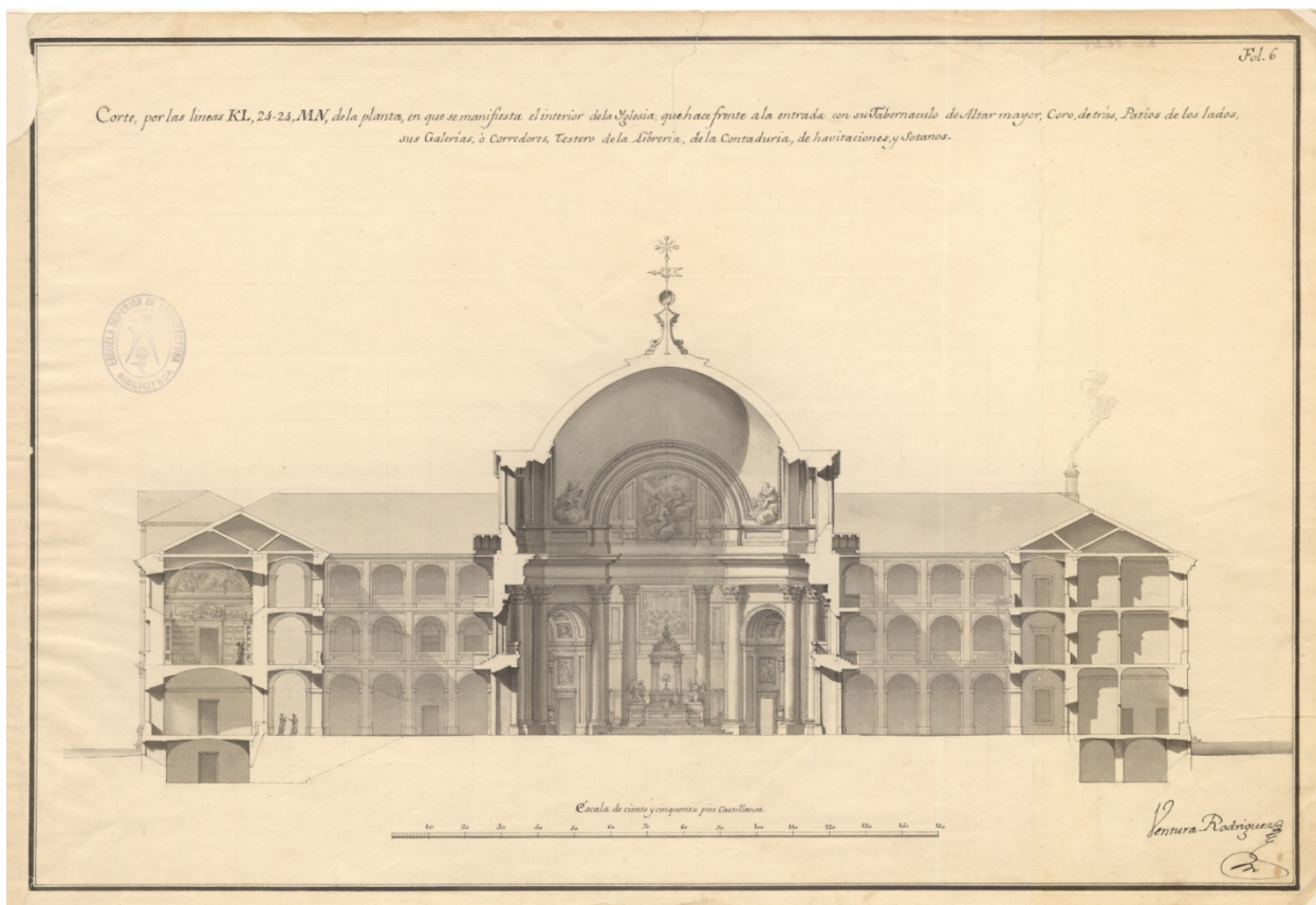
Fig. 39- Ventura Rodríguez: Sección "en que se manifiesta el interior de la Yglesia, que hace frente a la entrada con su Tabernáculo de Altar mayor, Coro detrás, Patios de los lados, sus Galerías o Corredores, Testero de la Librería, de la Contaduría, de habitaciones, y Sótanos", 1762. Escuela Técnica Superior de Arquitectura de Madrid.
