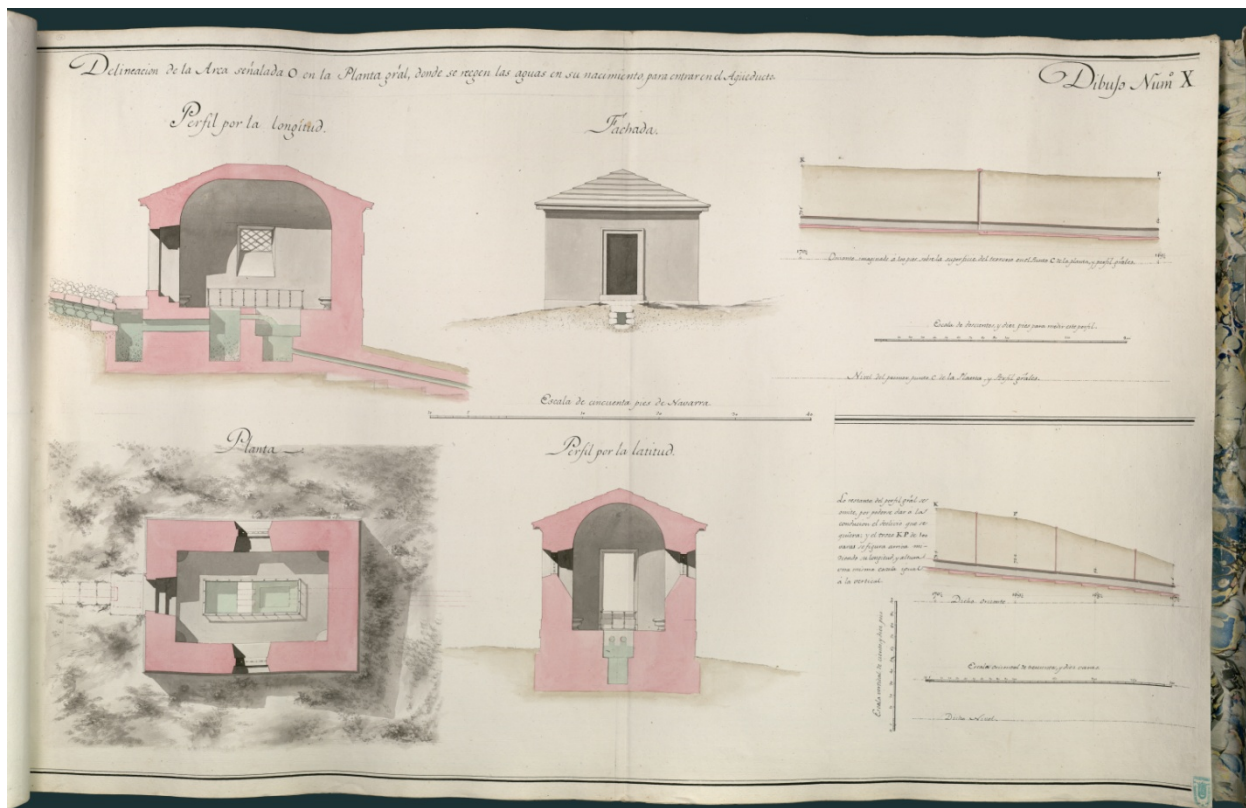
Fig. 100- Ventura Rodríguez: Delineación del acueducto de la ciudad de Pamplona, Dibujo Numº X , 1782. Archivo Municipal de Pamplona / Colección de Mapas, Planos y Dibujos.
