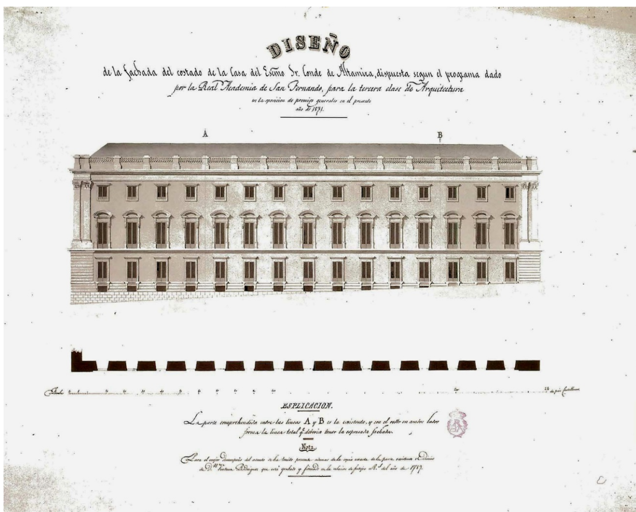
Fig. 211- Patricio de Velasco: Diseño de la fachada del costado de la Casa del Excmo. Sr. Conde de Altamira, dispuesta según el programa dado por la Real Academia de San Fernando, para la tercera clase de Arquitectura en la oposición de premios generales en el presente año de 1831 (primer premio). Real Academia de Bellas Artes de San Fernando.
