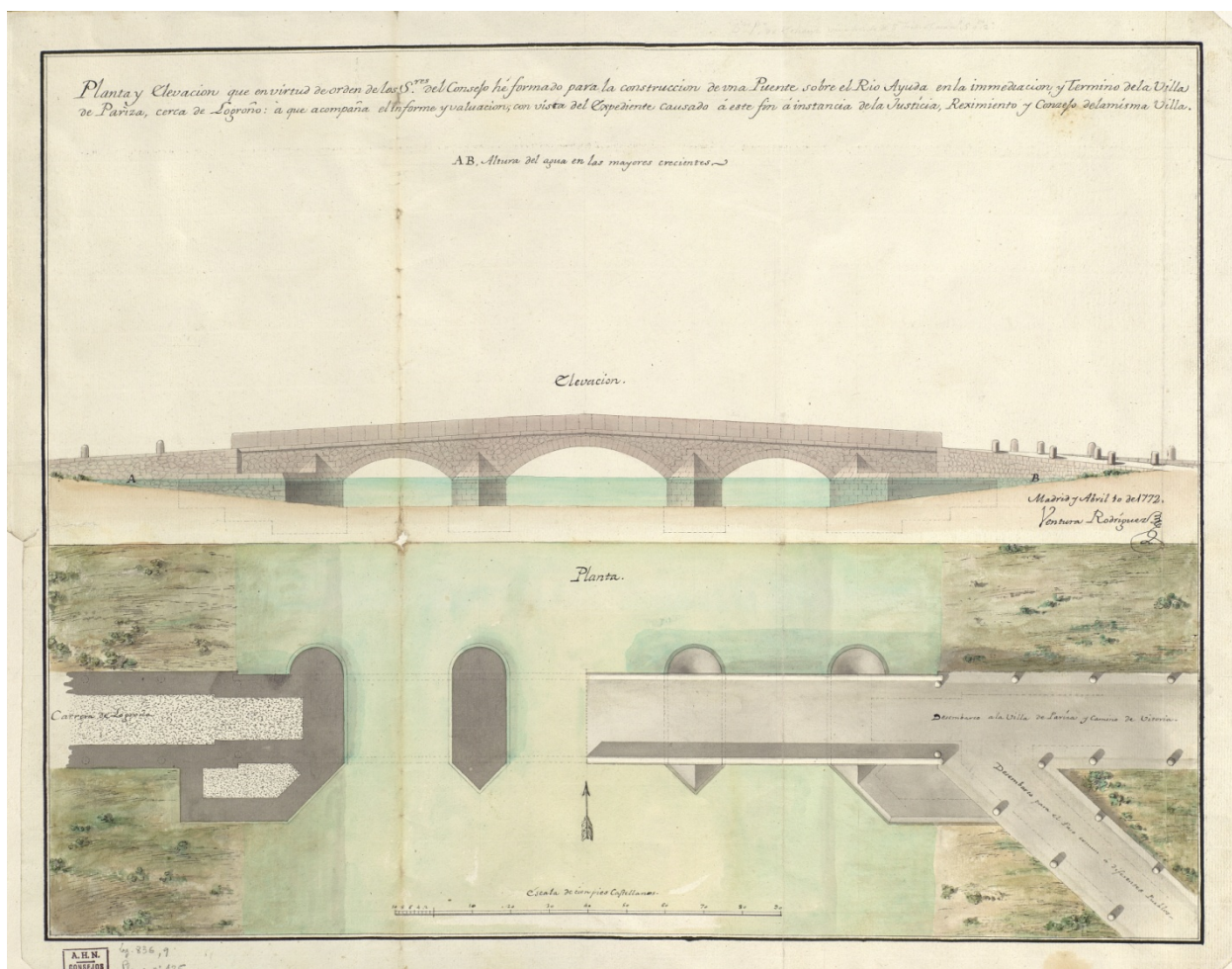
Fig. 121- Ventura Rodríguez: “Planta y elevación (...) para la construcción de una Puente sobre el río Ayuda en la inmediación y término de la Villa de Pariza, cerca de Logroño”, 1772. Archivo Histórico Nacional.
